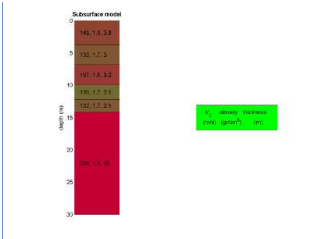
Figura 16: Indagine MASW2: Modello sismo stratigrafico
