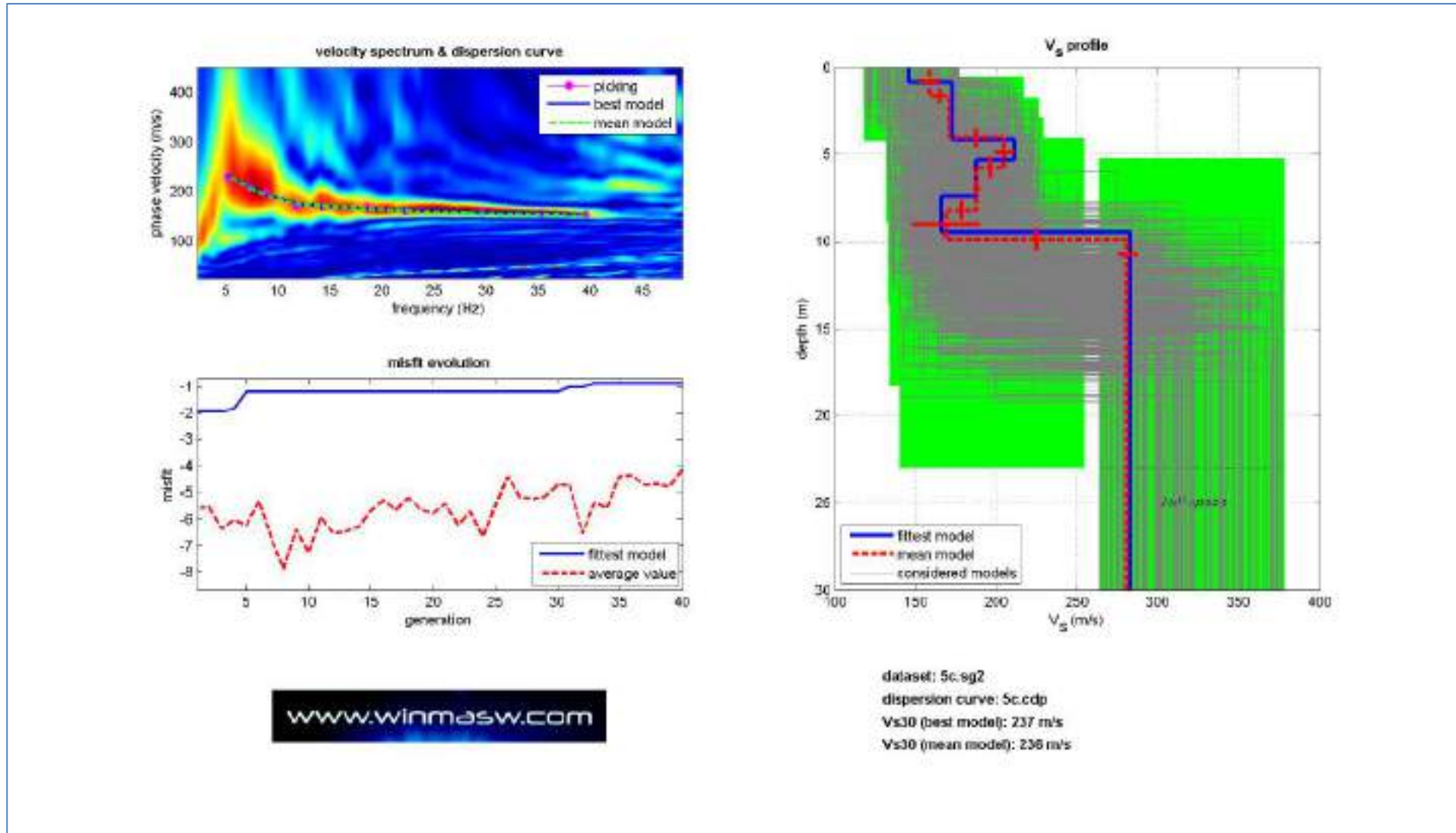
Figura 27: Indagine MASW6: Spettro osservato, curve di dispersione piccate e curve del modello individuato dall'inversione; profilo verticale V_s identificato; grafico misfit -generazione ( off-set 5m su G1 )
