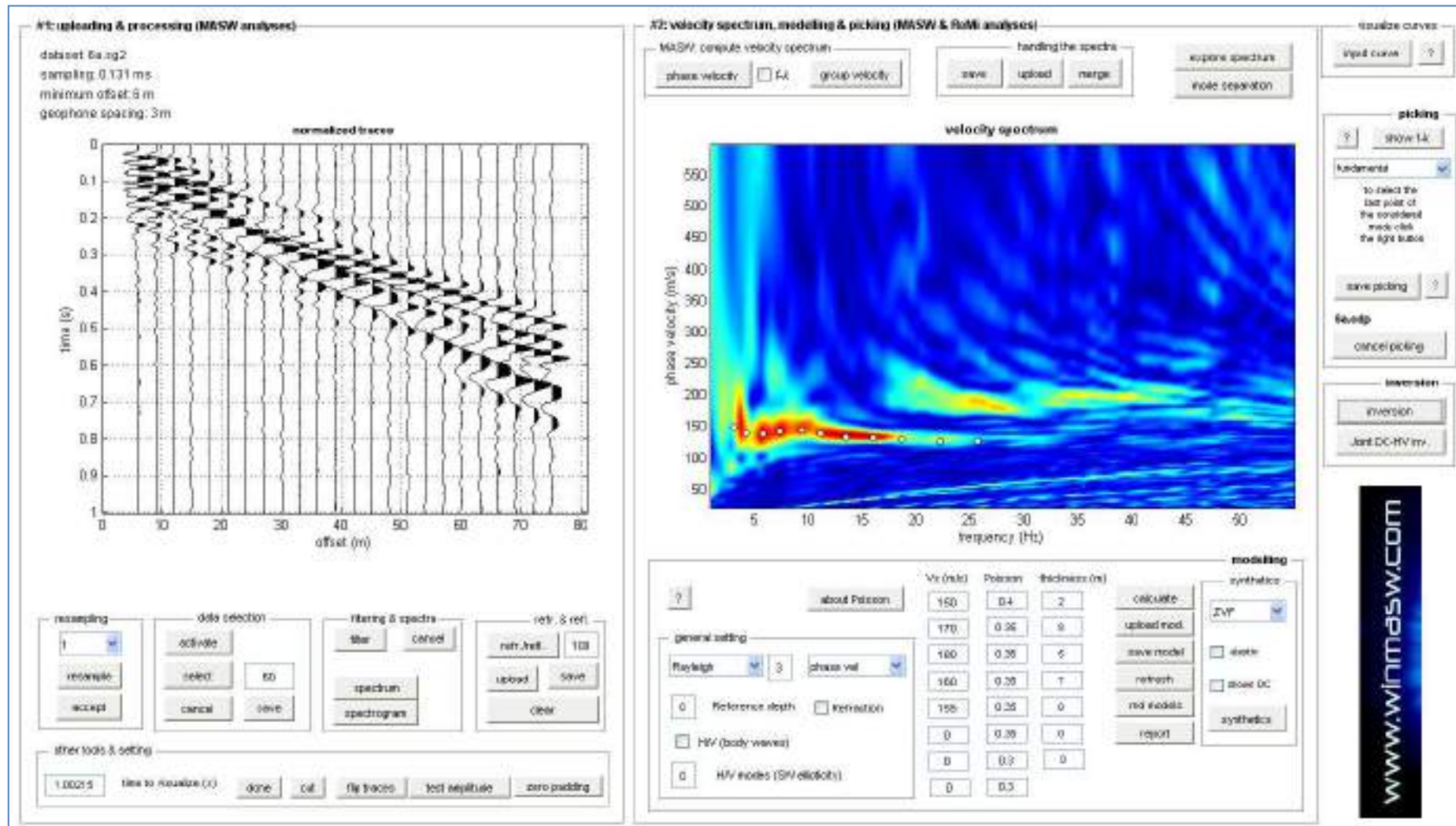
Figura 29: Indagine MASW7: Sismogramma, spettro di velocità; spettro e curva di dispersione individuata (picking) (off-set 6m su G1)
