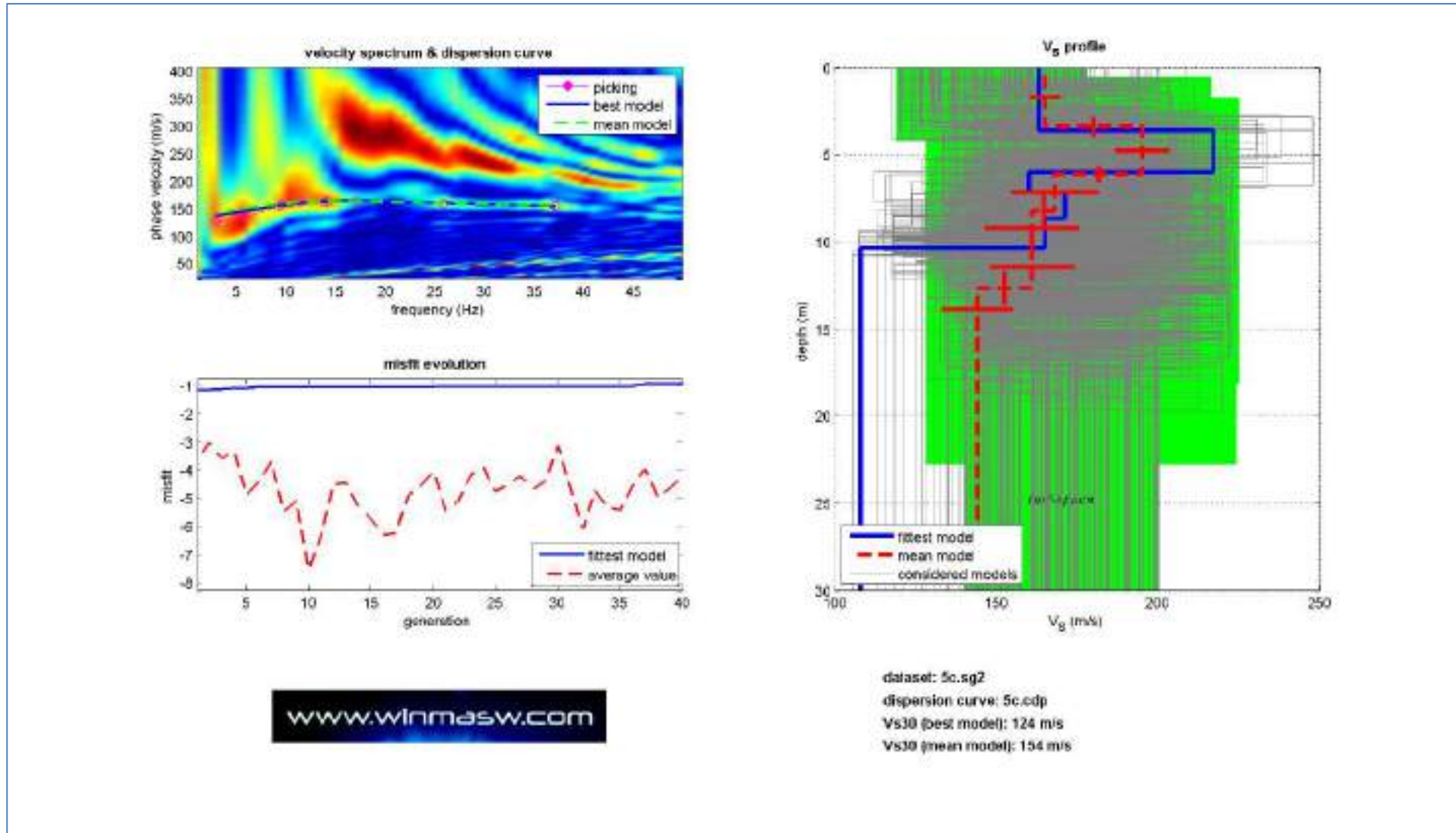
Figura 12: Indagine MASW1 : Spettro osservato, curve di dispersione piccate e curve del modello individuato dall'inversione; profilo verticale V_s identificato; grafico misfit -generazione ( off-set 5m su G1 )
