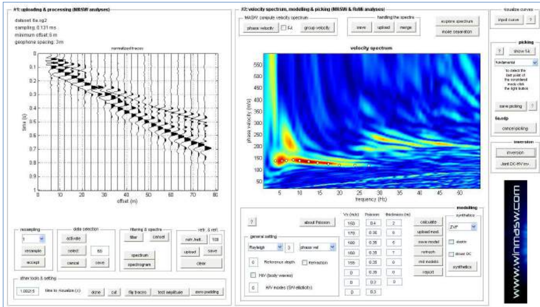
Figura 32: Indagine MASW8: Sismogramma, spettro di velocità; spettro e curva di dispersione individuata (picking) (off-set 6m su G1)
