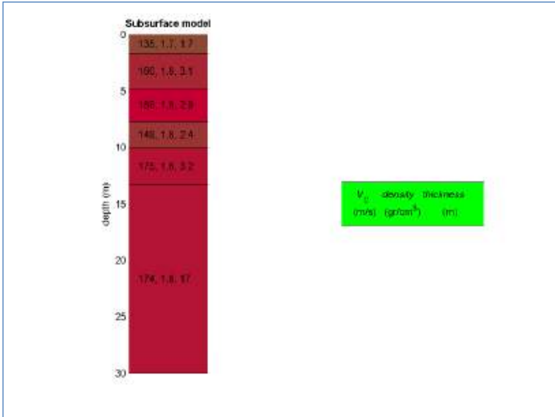
Figura 19: Indagine MASW3: Modello sismo stratigrafico
