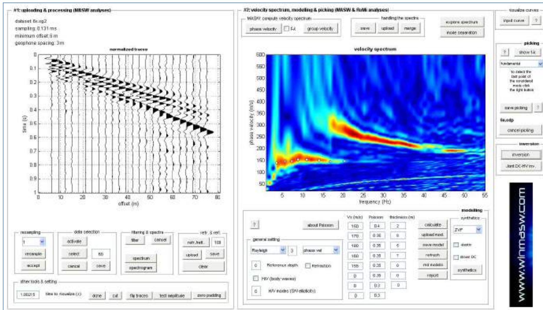
Figura 20: Indagine MASW4: Sismogramma, spettro di velocità; spettro e curva di dispersione individuata (picking) (off-set 6m su G1)
