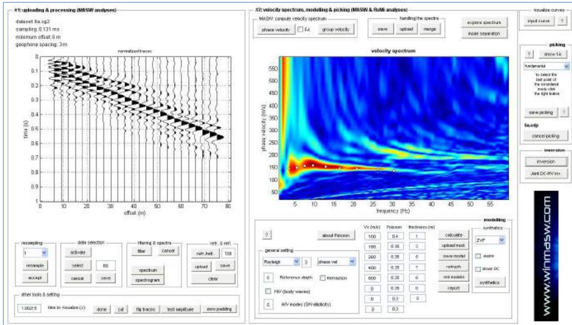
Figura 17: Indagine MASW3: Sismogramma, spettro di velocità; spettro e curva di dispersione individuata (picking) (off-set 6m su G1)
