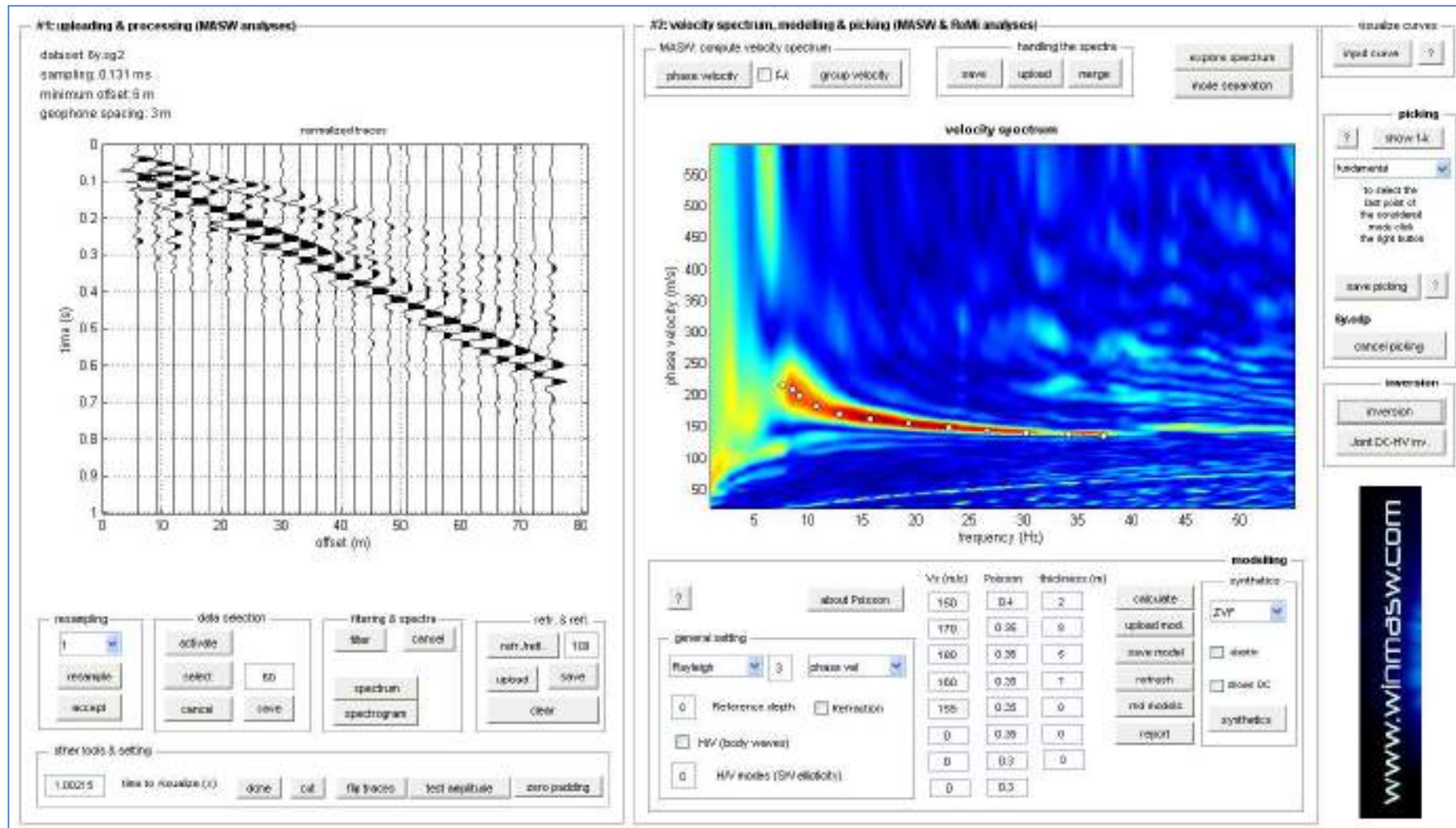
Figura 35: Indagine MASW9: Sismogramma, spettro di velocità; spettro e curva di dispersione individuata (picking) (off-set 6m su G1)
