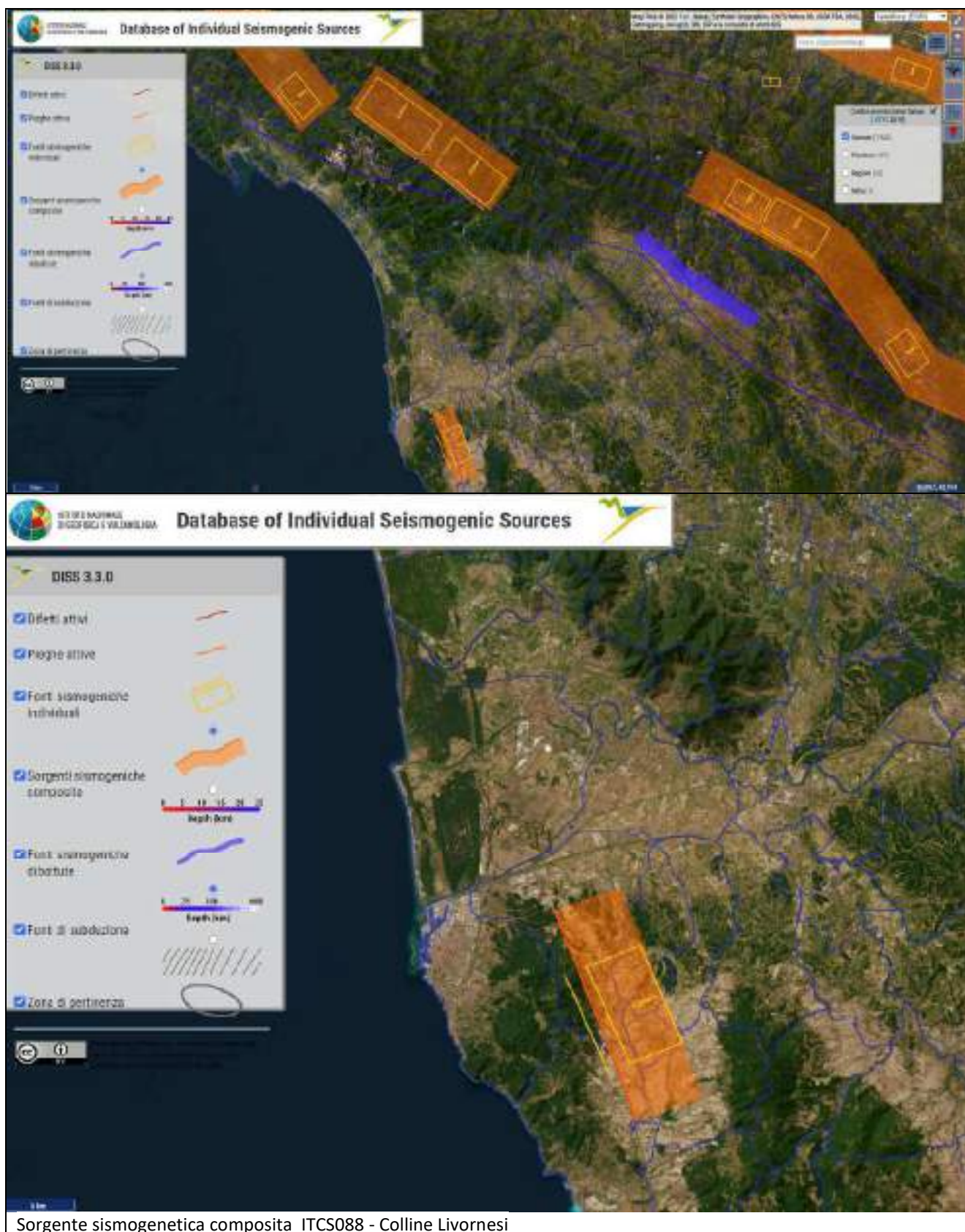
Fig.4.4 Fonti sismogenetiche (progetto DISS_3.3)
