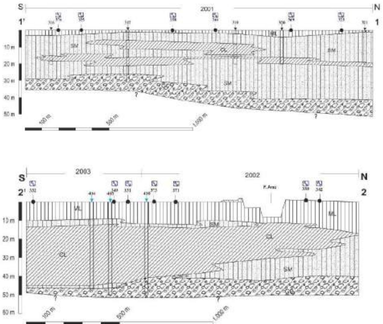
Fig.8.5 Sezioni -NS pianura territorio (Sardina-Oltrarno)
