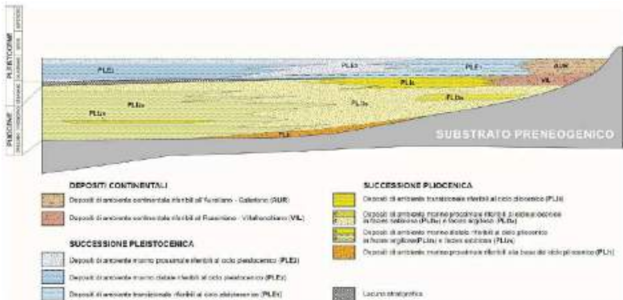
Fig.5.2 Rappresentazione schematica delle successioni stratigrafiche neogenico-quadernarie, (tratta da: Studio geologico-geomorfologico del PSI, pa.3,1 inquadramento geologico regionale )
