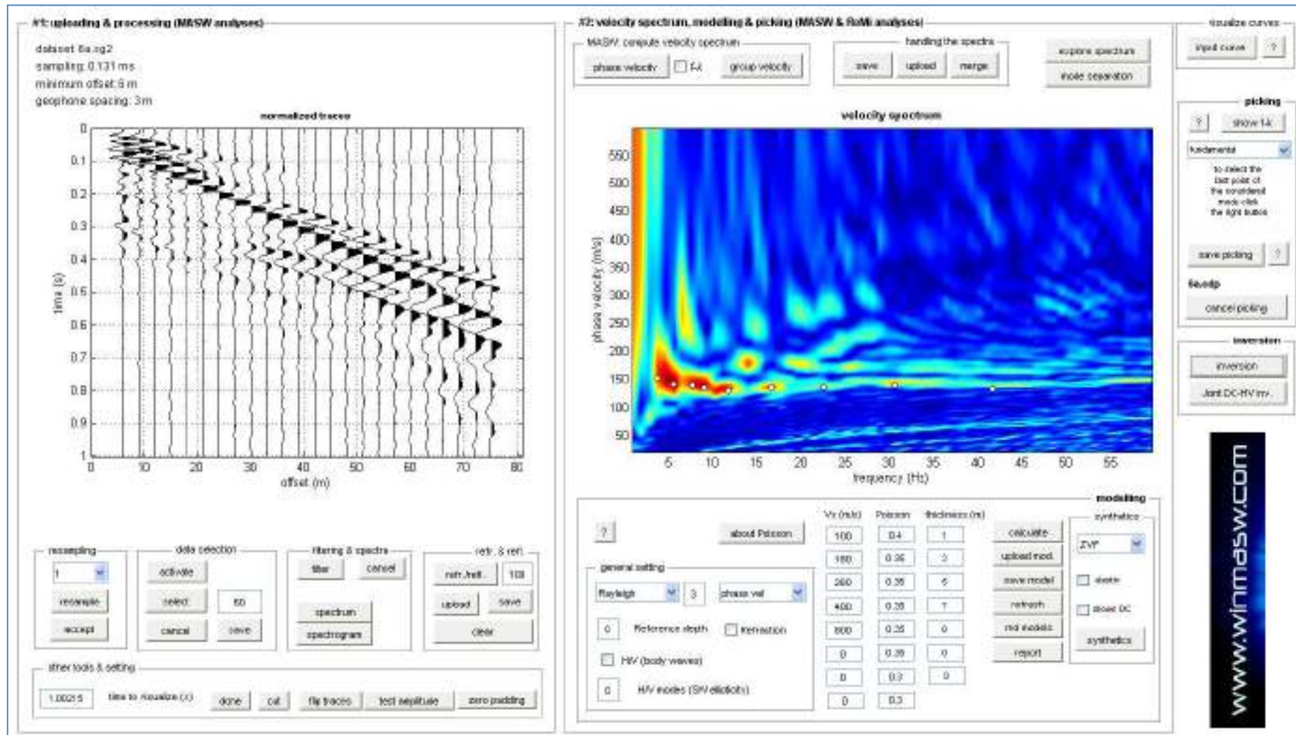
Figura 14: Indagine MASW2: Sismogramma, spettro di velocità; spettro e curva di dispersione individuata (picking) (off-set 6m su G1)
