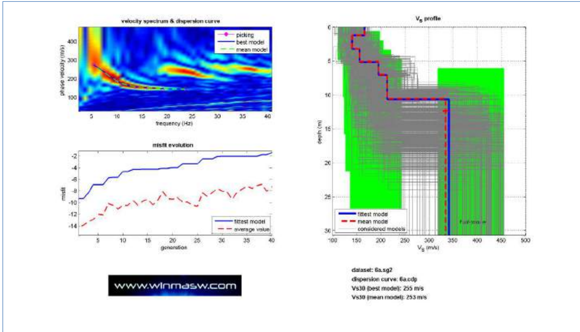
Figura 24: Indagine MASW5 : Spettro osservato, curve di dispersione piccate e curve del modello individuato dall'inversione; profilo verticale V_s identificato; grafico misfit-generazione ( off-set 6m su G1 )
