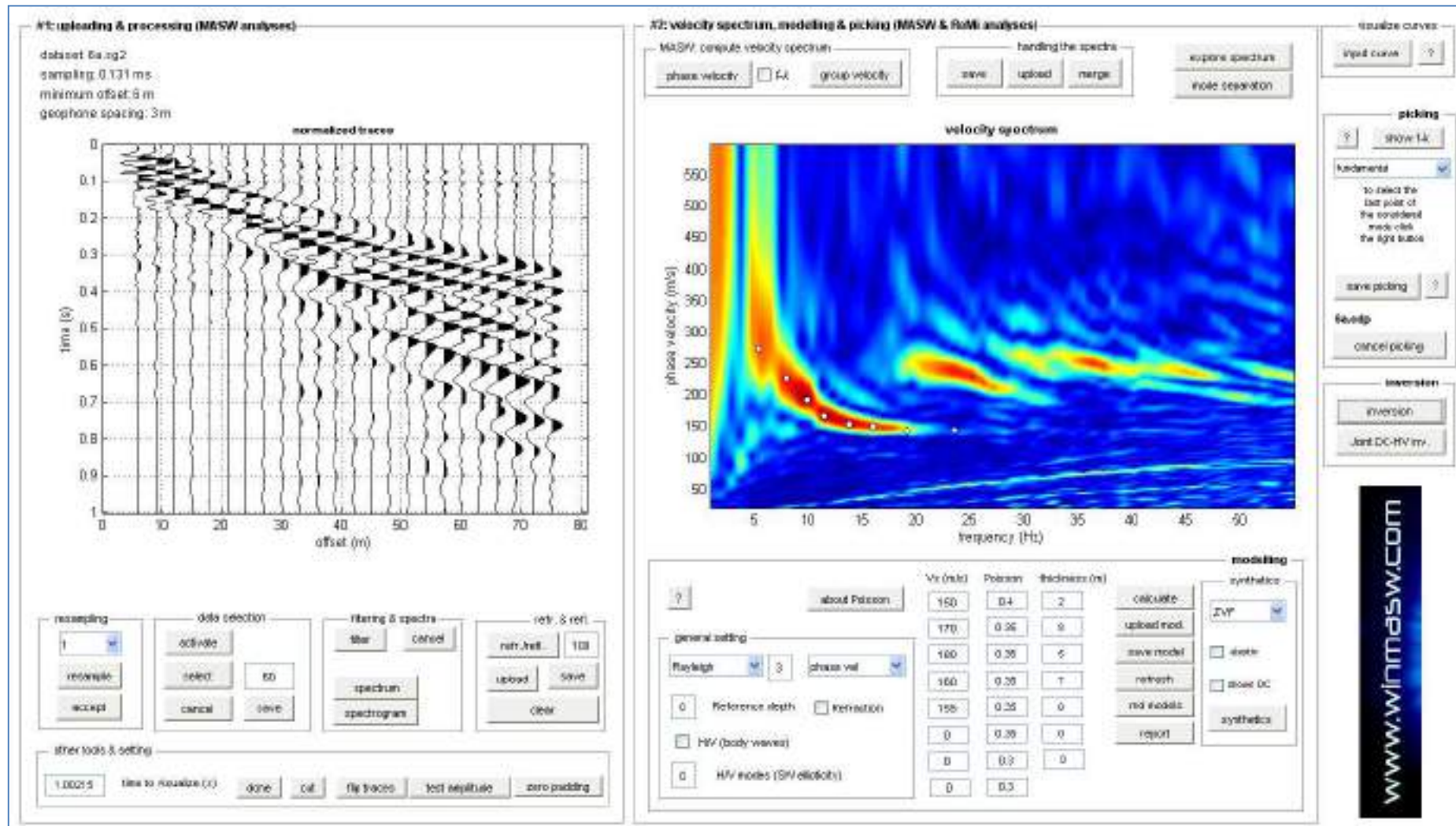
Figura 23: Indagine MASW5: Sismogramma, spettro di velocità; spettro e curva di dispersione individuata (picking) (off-set 6m su G1)
