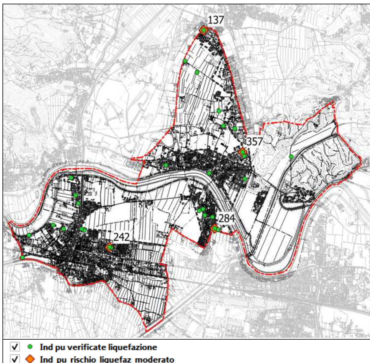
Fig.9.3 Distribuzione prove CPT/CPTU di verifica a liquefazione
