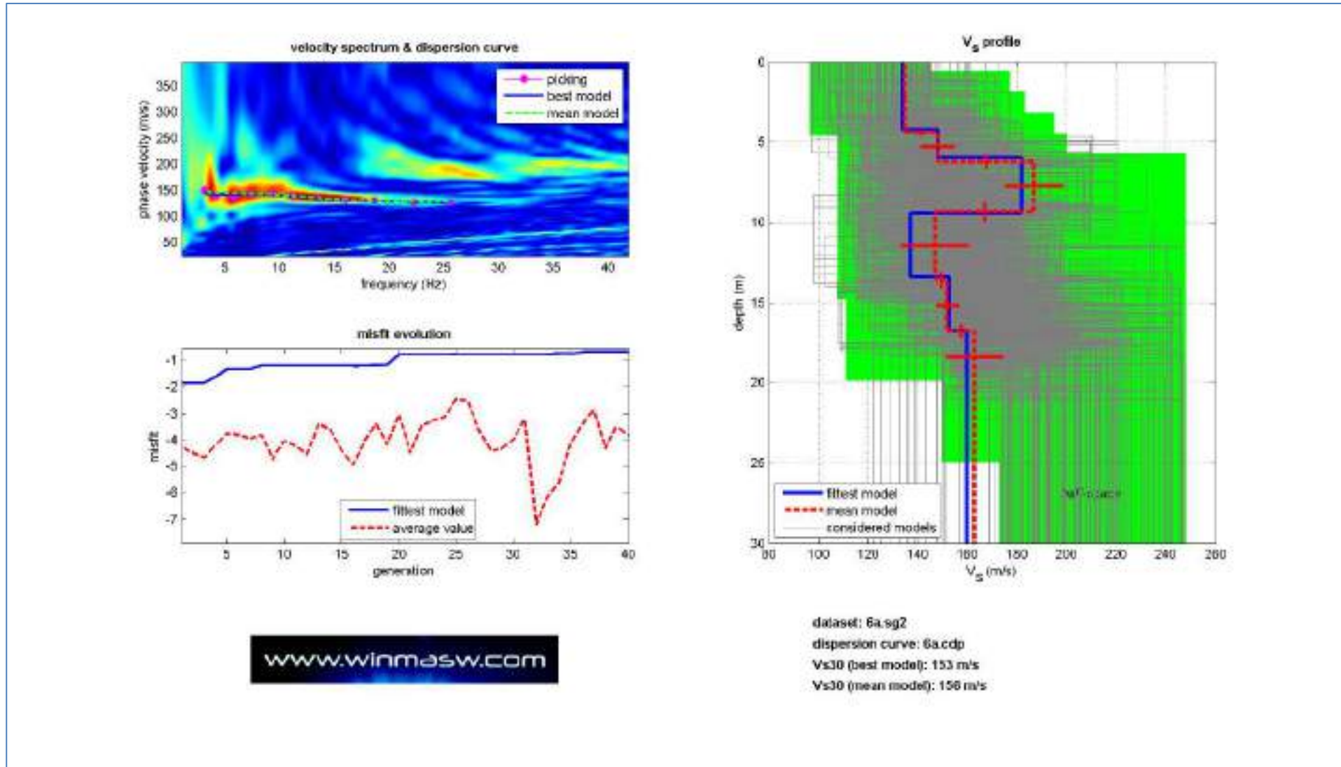
Figura 30: Indagine MASW7: Spettro osservato, curve di dispersione piccate e curve del modello individuato dall'inversione; profilo verticale V_s identificato; grafico misfit -generazione ( off-set 6m su G1 )
