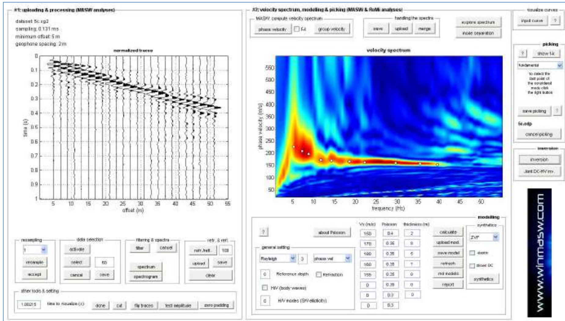
Figura 26: Indagine MASW6: Sismogramma, spettro di velocità; spettro e curva di dispersione individuata (picking) (off-set 5m su G1)
