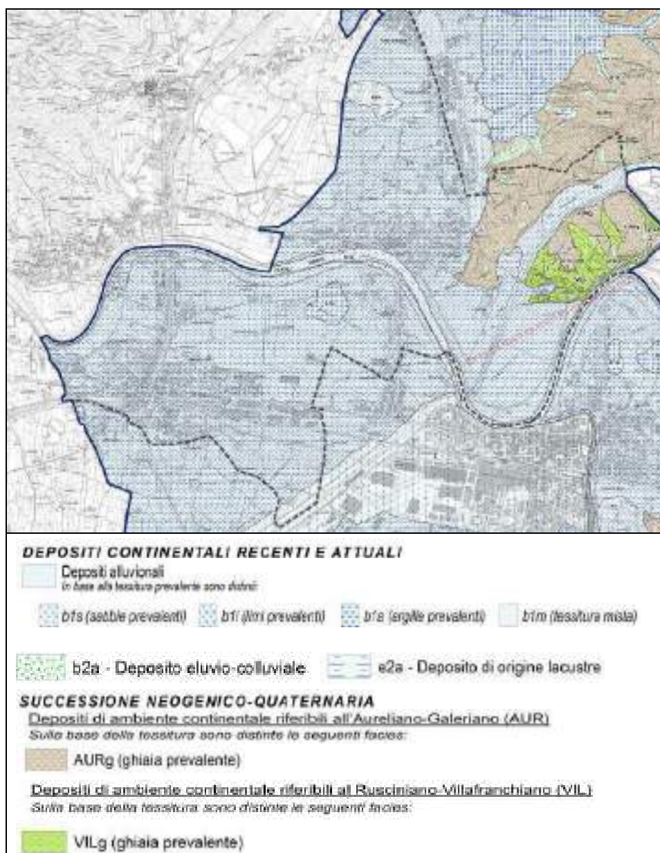
Fig.5.1 Carta Geologica PSI adottata e modificata a seguito osservazioni
