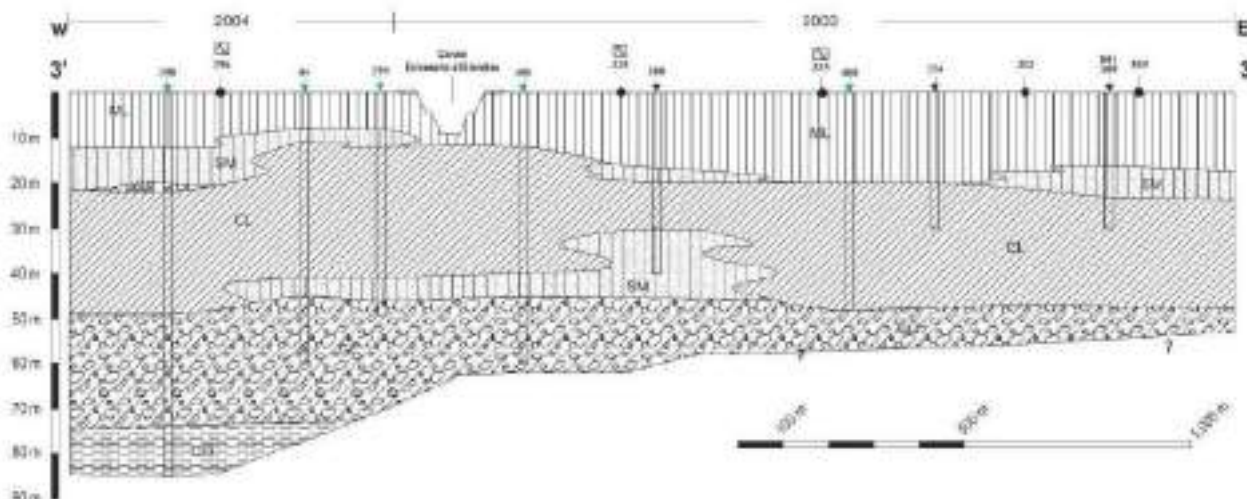
Fig.8.6 Sezione E-W pianura territorio comune (Fornacette)
