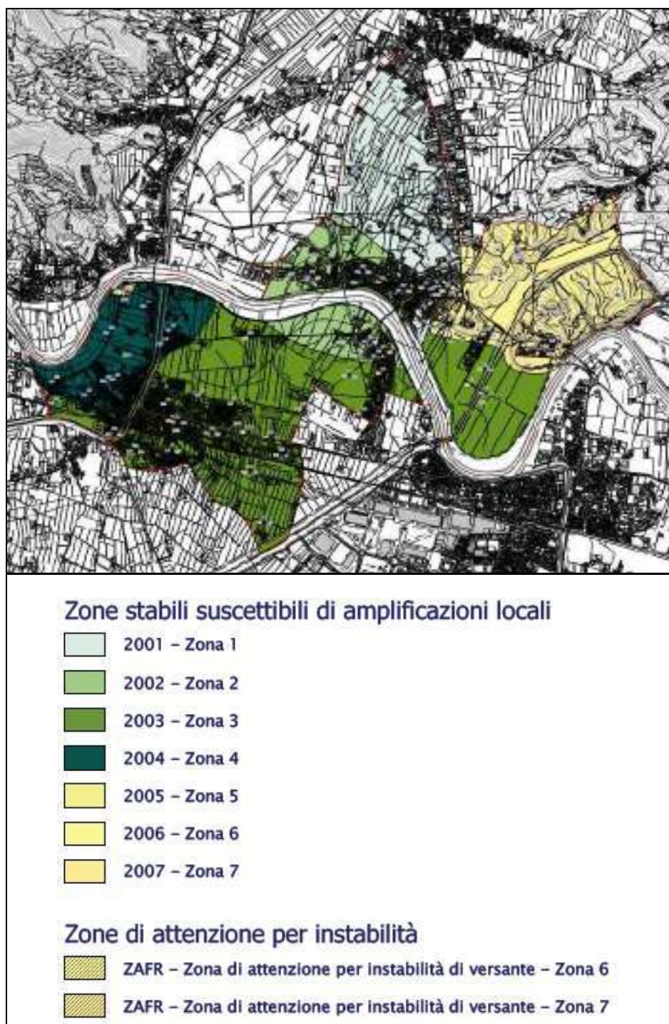
Fig.9.1 Carta delle MOPS MS2 (revisione livello1)
