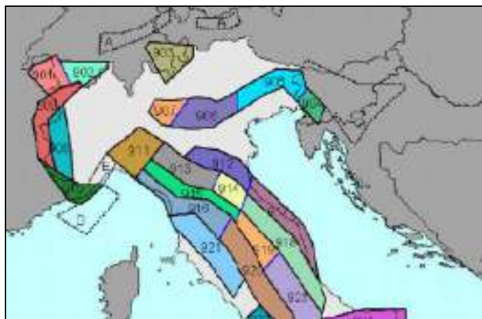
Fig.4.2 Carta della sismicità
