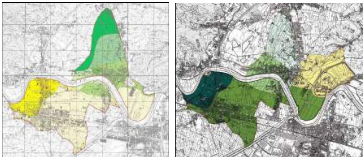
Fig.9.2 Raffronto Carte MOPS MS1 (sx) e MS2 (dx)
