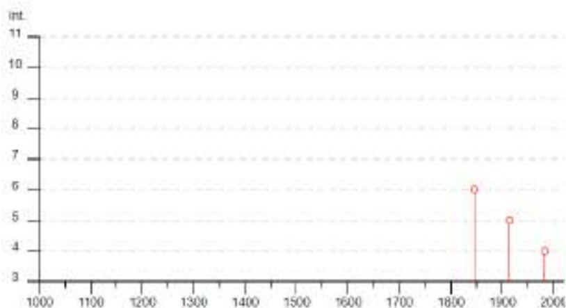
Fig.4.7 Storia sismica di Calcinai come risulta dal DataBase Macrosismico Italiano, DBMI15 ( https://emidius.mi.ingv.it/CPTI15-DBMI15 )
