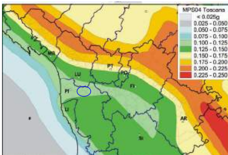
Fig.4.1 Classificazione sismica regionale
